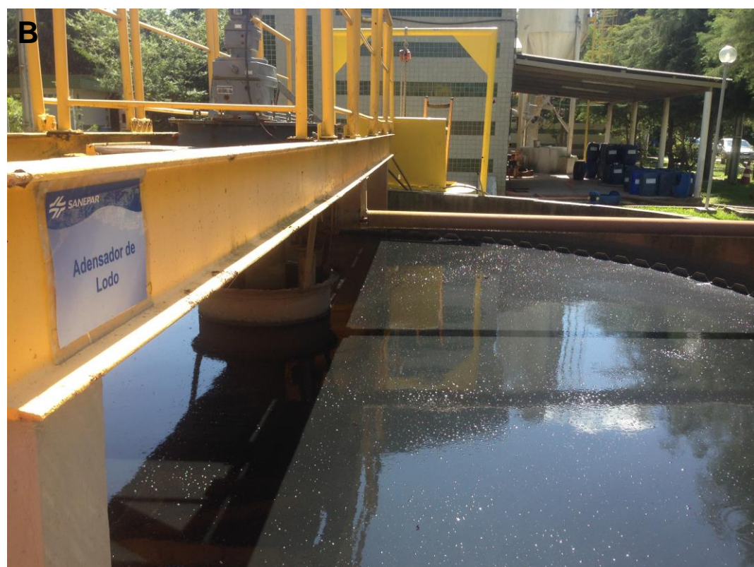
Figura 4.6. Vistas da Estação de Tratamento de Esgoto Santa Quitéria, no Município de Curitiba-PR em maio de 2016, onde ocorre tratamento da maior parte do esgoto domiciliar coletado através de “rede geral de esgoto ou pluvial”: tanques (A) e adensador de lodo (B).
