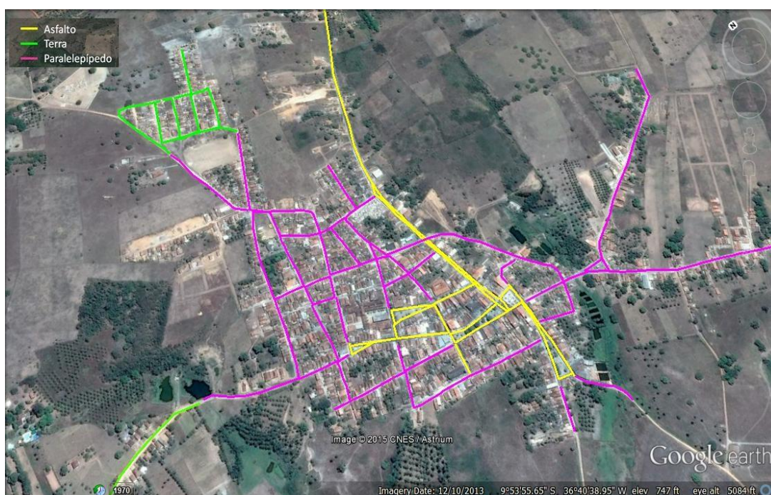
Figura 13: Sistema viário da área urbana por tipo de revestimento
