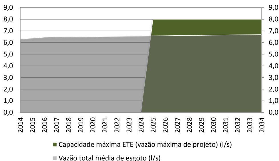
Figura 11: Projeção de demanda SES – Cenário Tendencial – Sede Fonte: Gesois, 2015.
