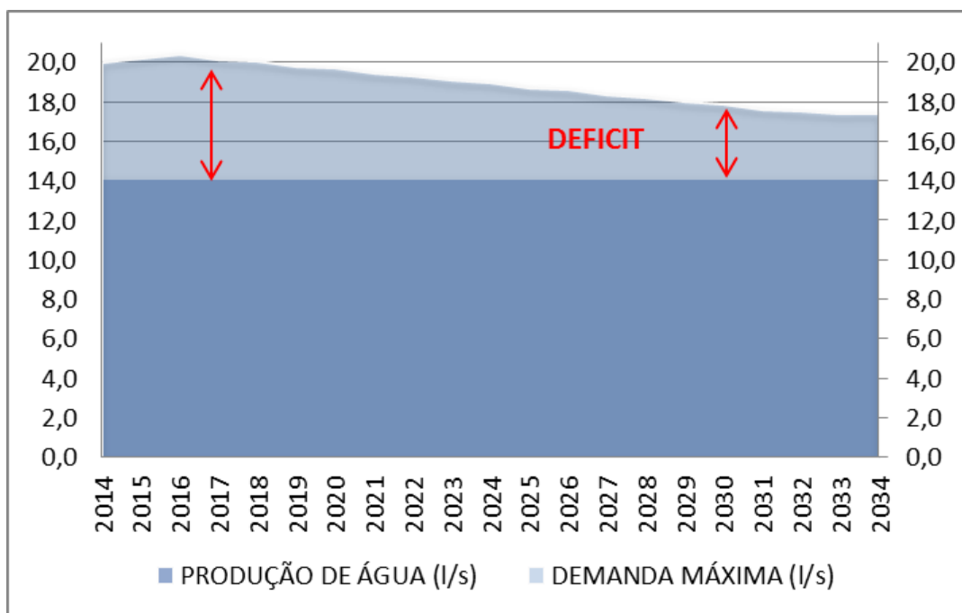
Figura 8: Projeção de demanda SAA - Cenário Tendencial - CASAL Fonte: Gesois, 2014.
