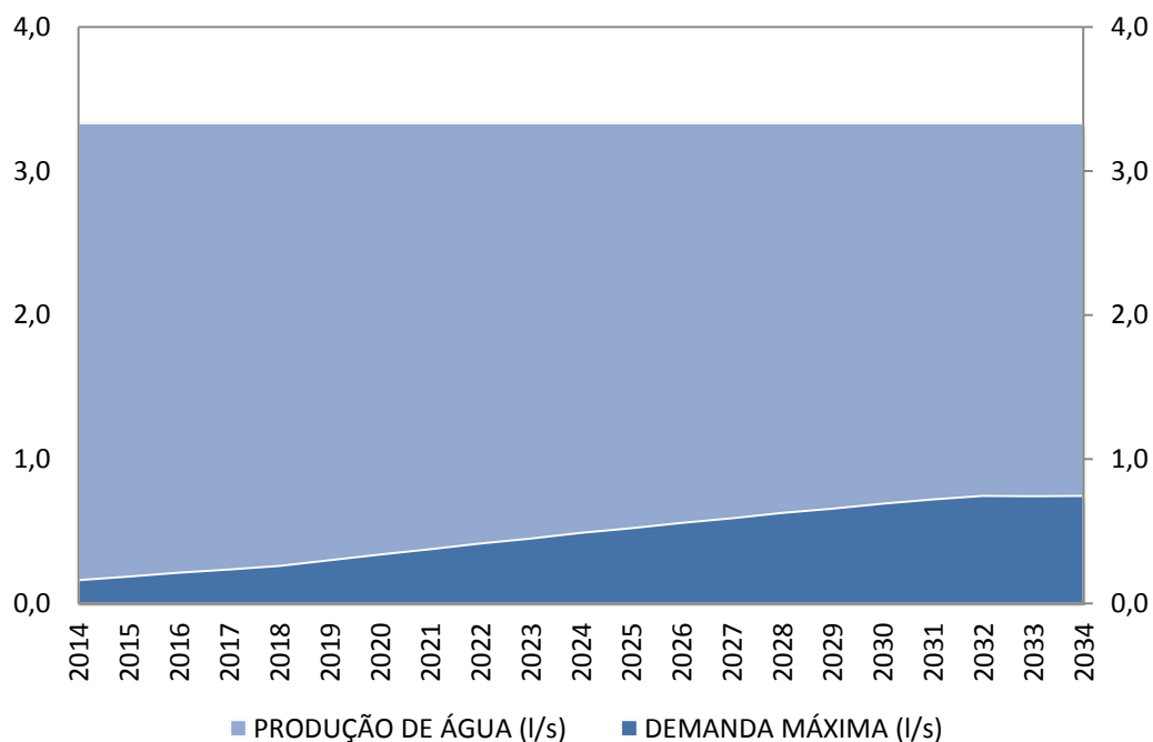
Figura 9: Projeção de demanda SAA - Cenário Tendencial – Prefeitura (Povoado de Varzinha)
