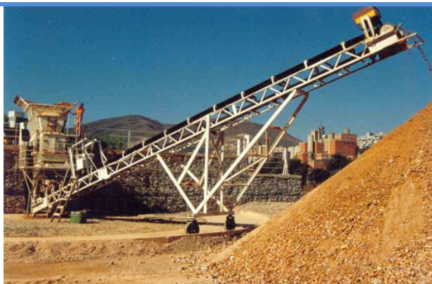
Figura 36: Usina de reciclagem de entulho da Construção Civil Fonte: SLU/CEMP, 2013.
