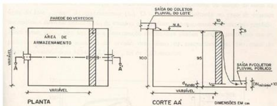
Figura 53: Esquema de um microrreservatório Fonte: A. JÚNIOR (2008).
