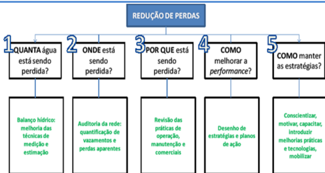
Figura 12: Modelo de avaliação e controle de perdas em sistemas de abastecimento de água
