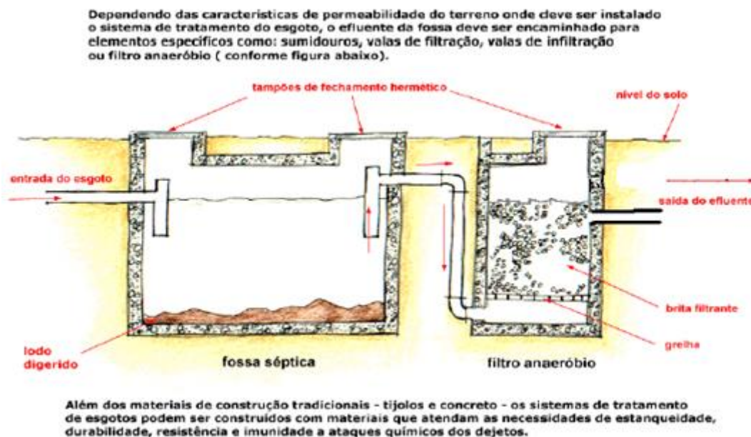
Figura 30: Conjunto fossa séptica – filtro anaeróbio Fonte: Edifique, 1999.
