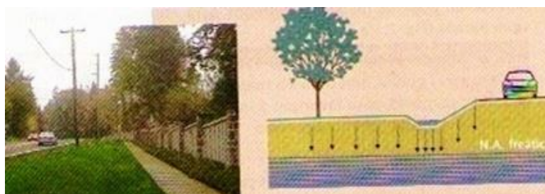
Figura 44: Vala de infiltração Fonte: PROSAB, 2009.
