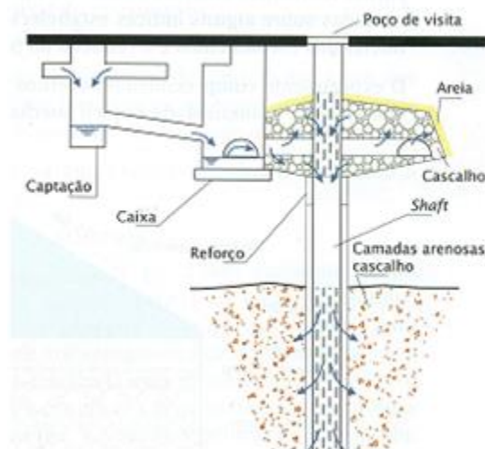
Figura 50: Estrutura típica de um poço de infiltração Fonte: Canholi, 2005.
