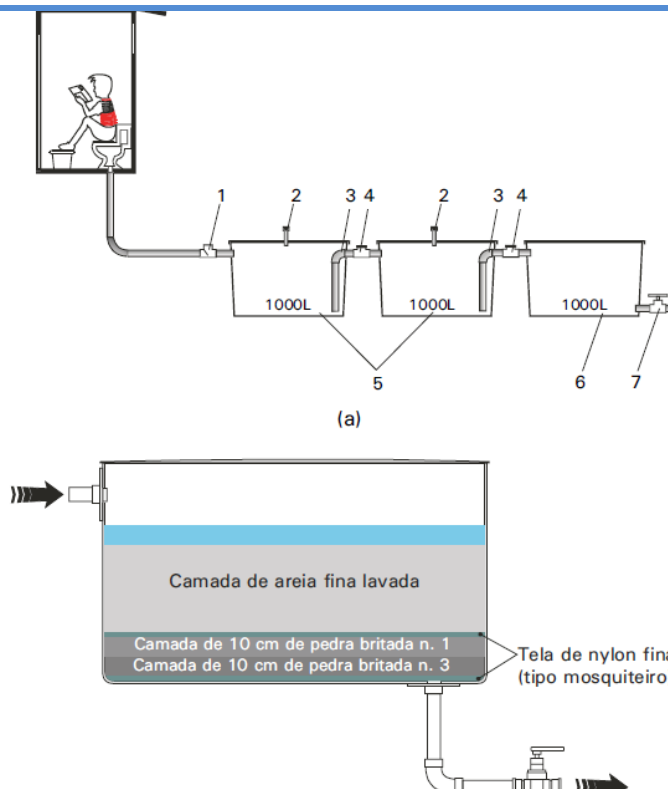
Figura 28: Esquema de um Biodigester Fonte: Embrapa, 2010.
