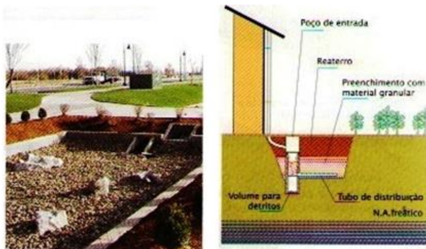
Figura 47: Bacia de percolação
