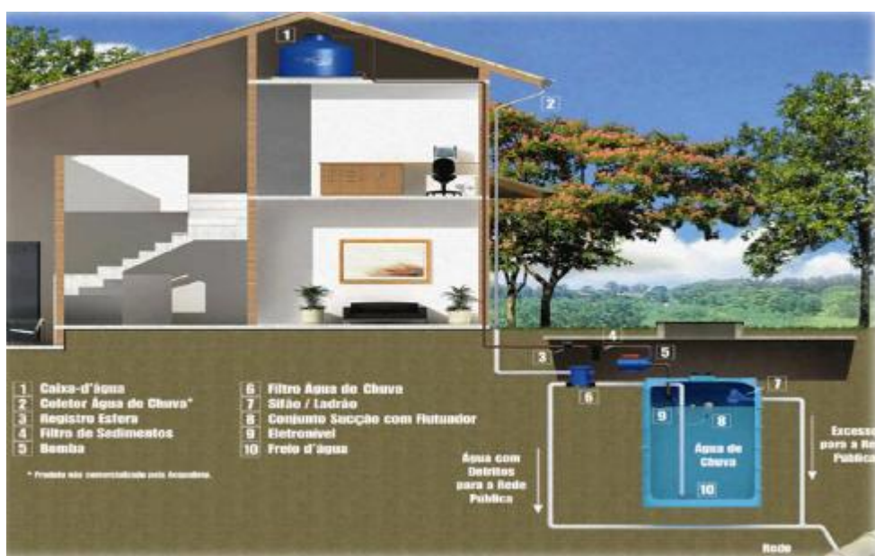
Figura 17: Esquema de captação de água de chuva
