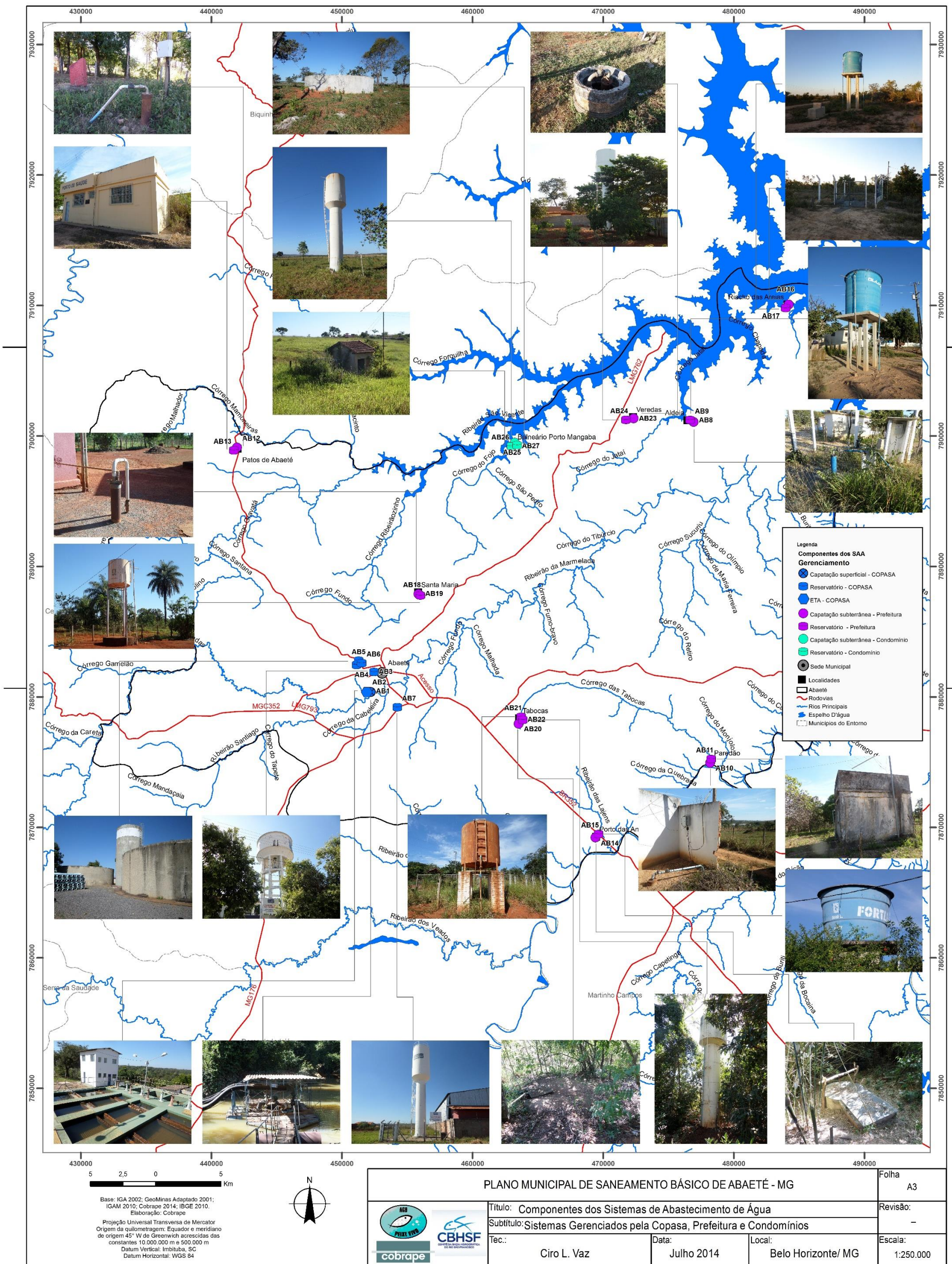
Figura 9.1 – Componentes dos sistemas de abastecimento de água do município de Abaeté
