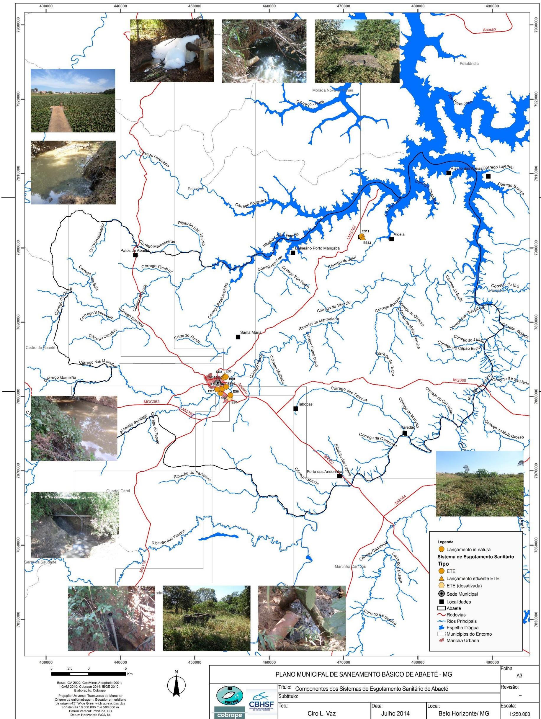
Figura 9.2 – Principais componentes dos sistemas de esgotamento sanitário da sede do município de Abaeté
